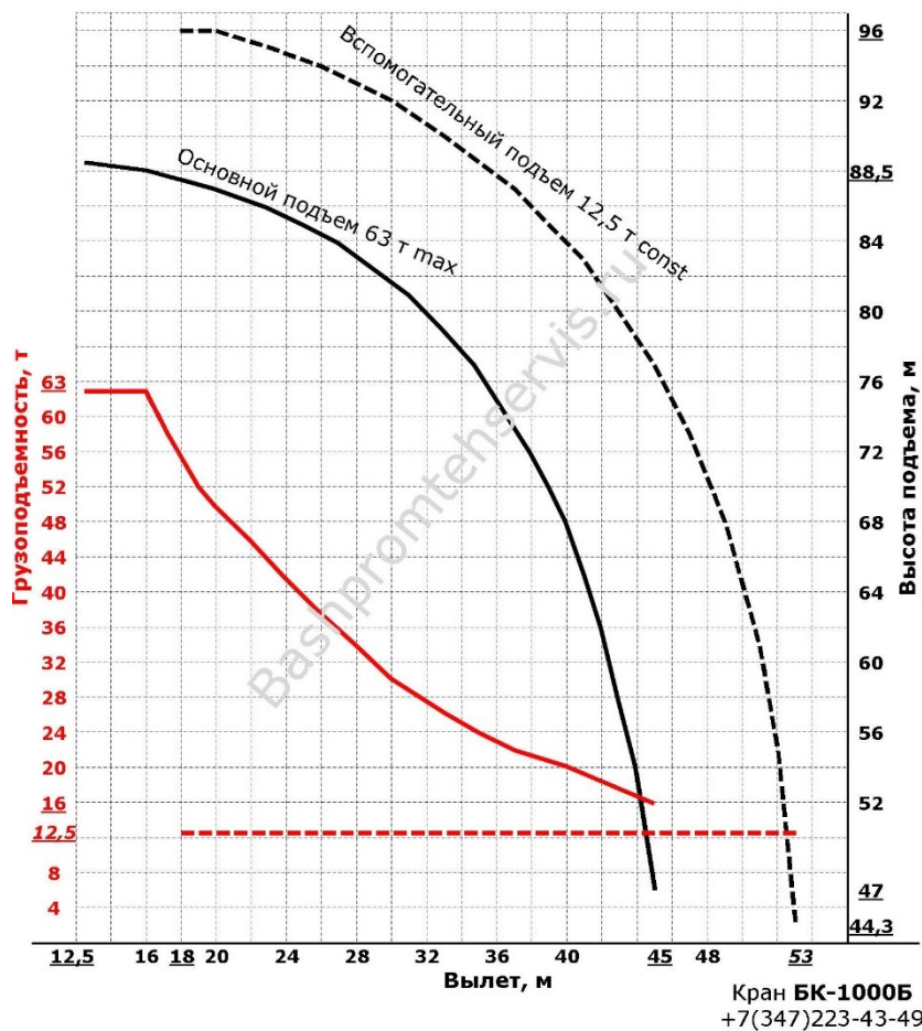
Рис. 2. Грузовысотные характеристики крана БК-1000Б
