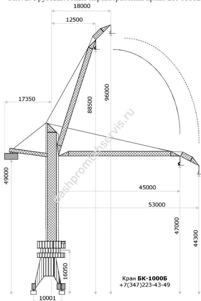
Рис. 1. Схема крана БК-1000Б (заводская комплектация, возможно увеличение высоты подъема).
